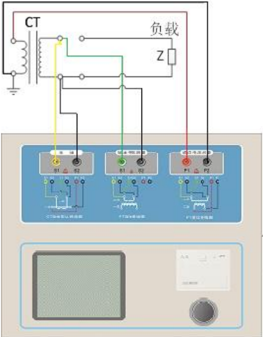
图2.1 CT直阻、励磁、变比试验接线方式
