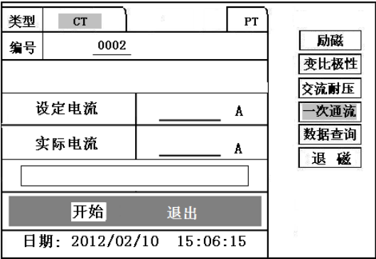
图 14、CT 一次通流测试界面
