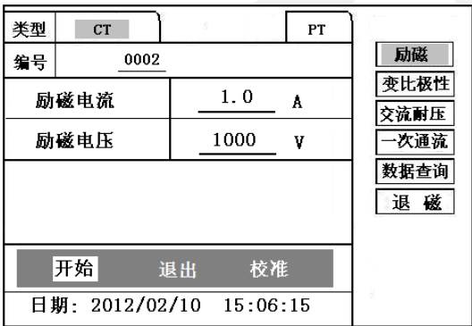
图 4，CT 励磁特性测试界面
