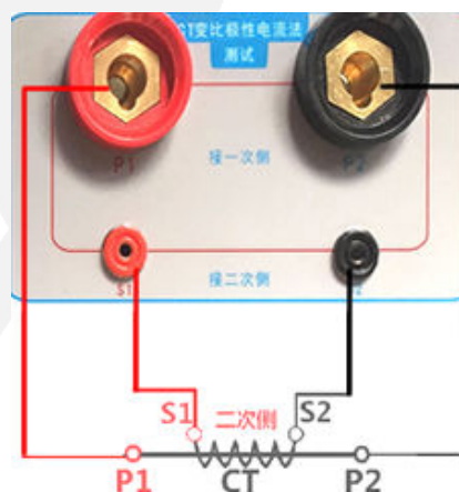
图 13 , CT 变比极性接线图
