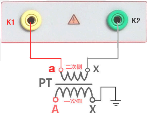
图 19，PT 励磁特性接线
